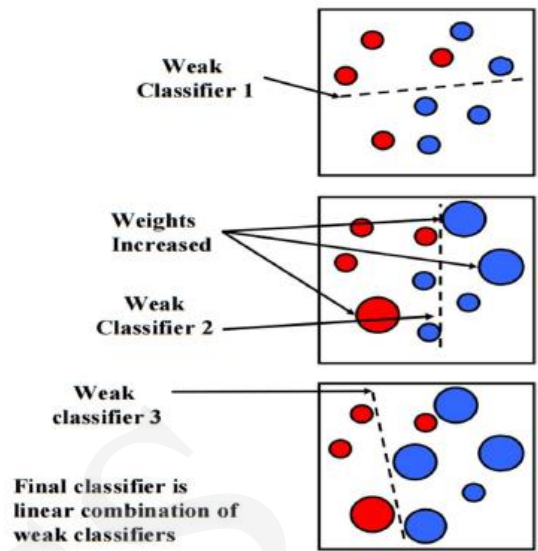
Fig. 3 AdaBoost[4]
