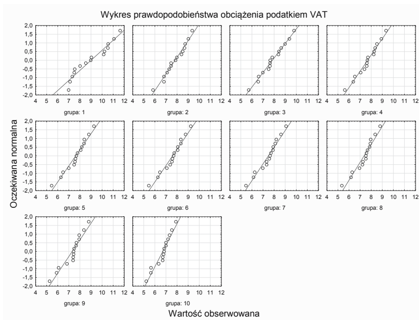
Rysunek. 1. Skatyzowane wykresy normalności
