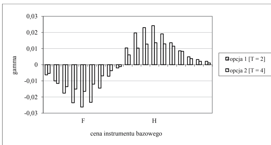
Rysunek 3. Wpływ ceny instrumentu bazowego oraz terminu wygaśnięcia na kształtowanie się wartości współczynnika gamma ceny korytarzowych opcji kupna
