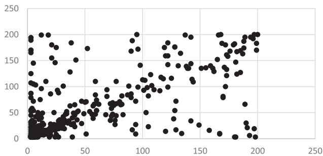
Rysunek 3. Zależności między długościami średnich ruchomych SMA I (oś odciętych) i EMA I (oś rzędnych) dla wszystkich analizowanych spółek
